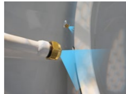
Buses de nettoyage pour sortie de cuve
