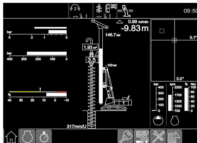
Pantalla para perforación con barrena continua
