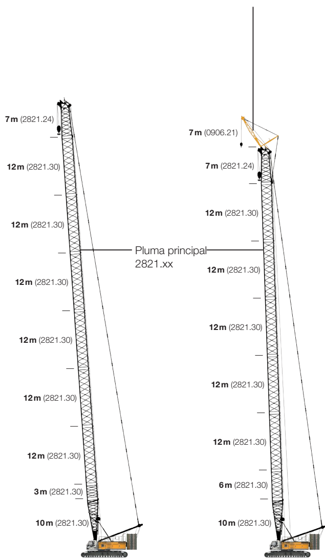
Plumín fijo 0906.21
